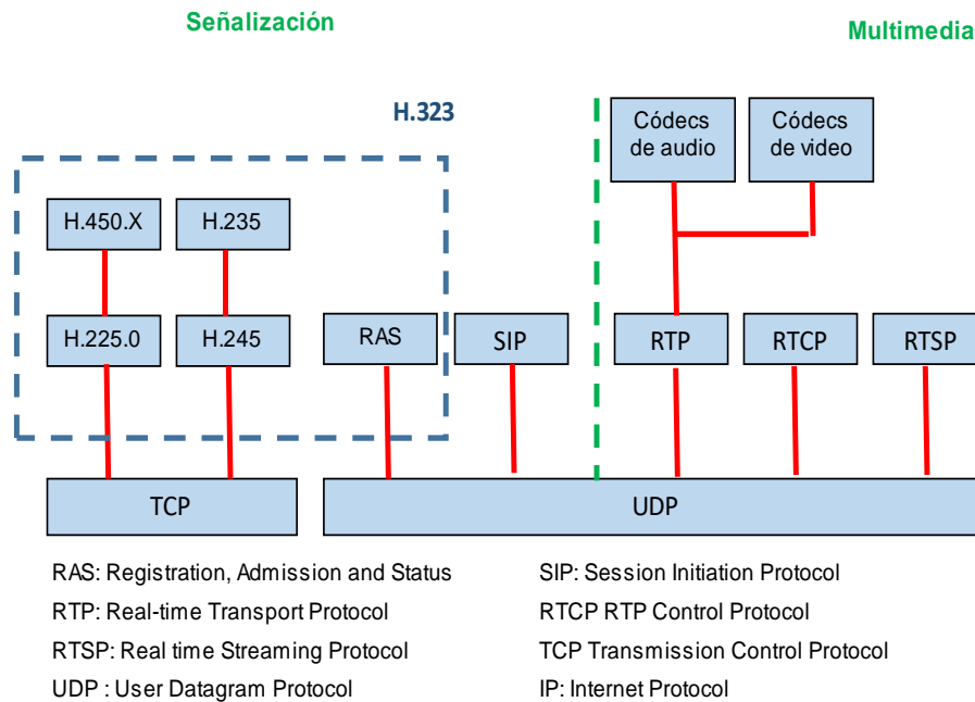
Figura 2: Estructura protocolo de VoIP
