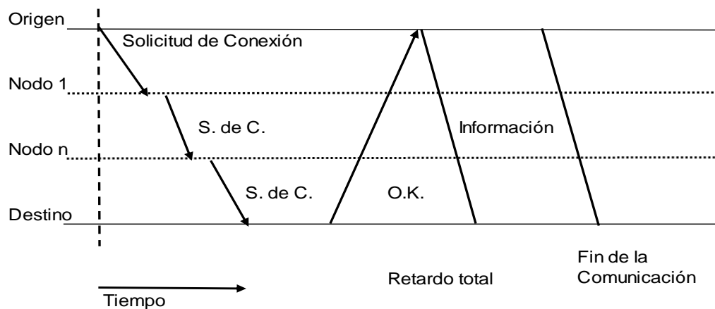
Figura N.º 01: Técnicas de conmutación de circuitos.
