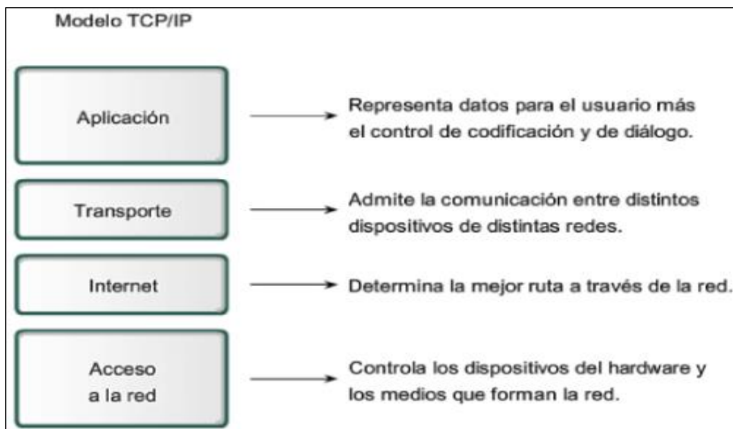
Figura 2: Modelo TCP/IP
