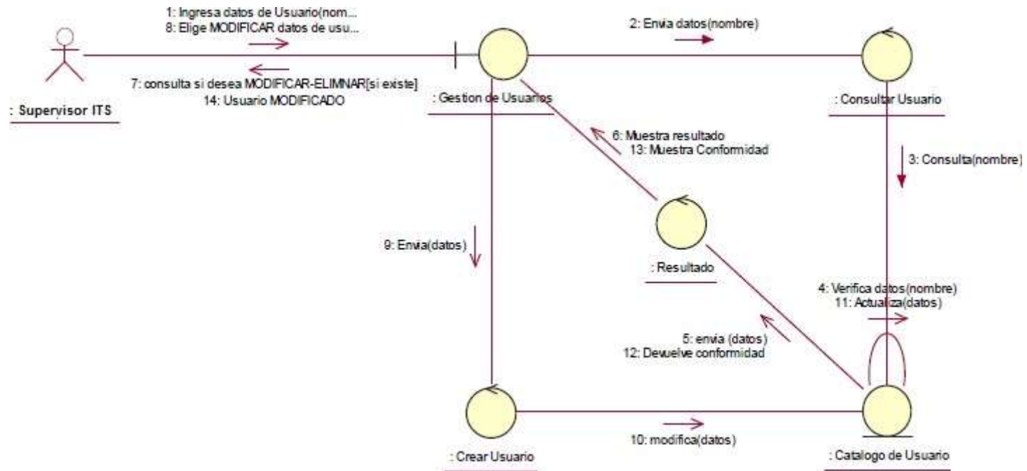
3.9.1.2. Figura N-° 13: Caso de uso: Modificar usuario.
