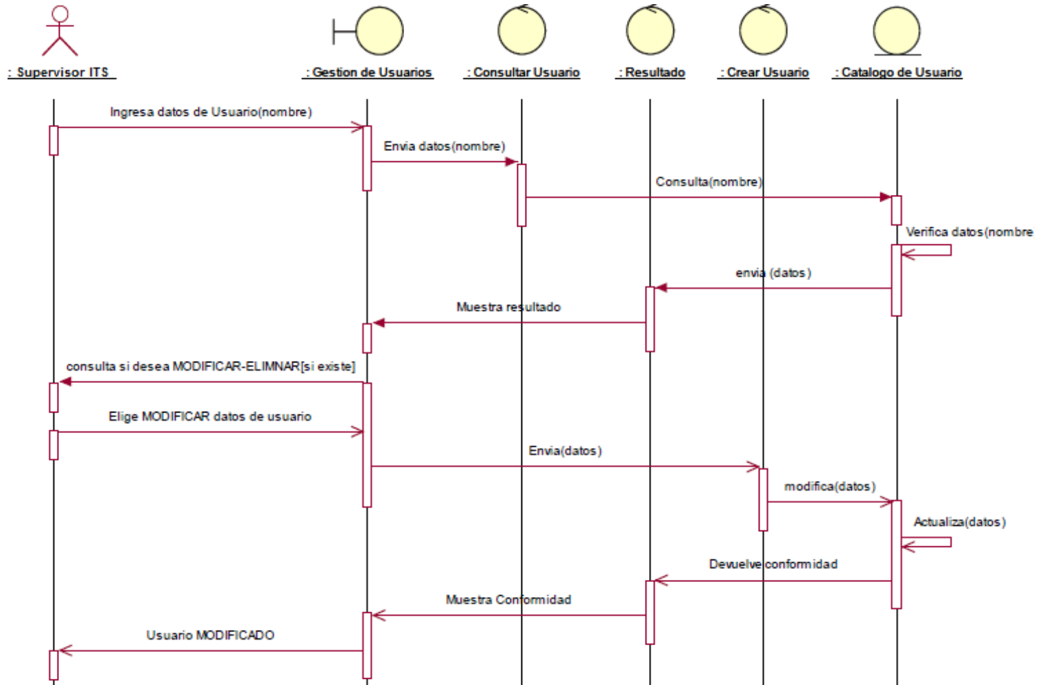
3.9.2.2. Figura N-° 26: Caso de uso: Modificar usuario.
