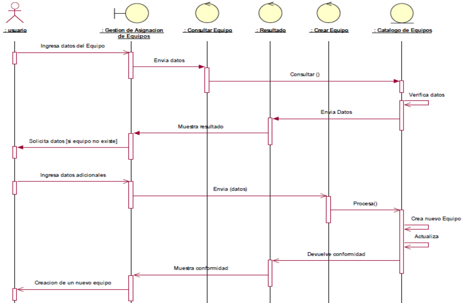
3.9.2.5. Figura N-º 29: Caso de uso: Registrar equipo.
