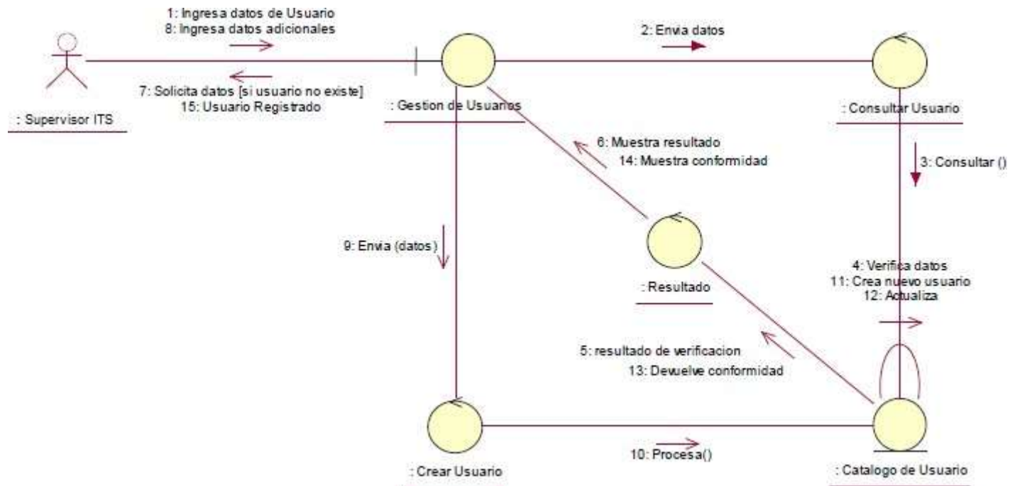
3.9.1.1. Figura N-º 12: Caso de uso: Registrar usuario.
