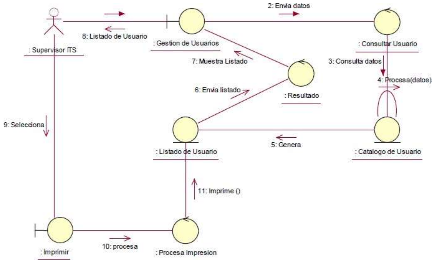
3.9.1.4. Figura N-º 15: Caso de uso: Reporte de usuarios.
