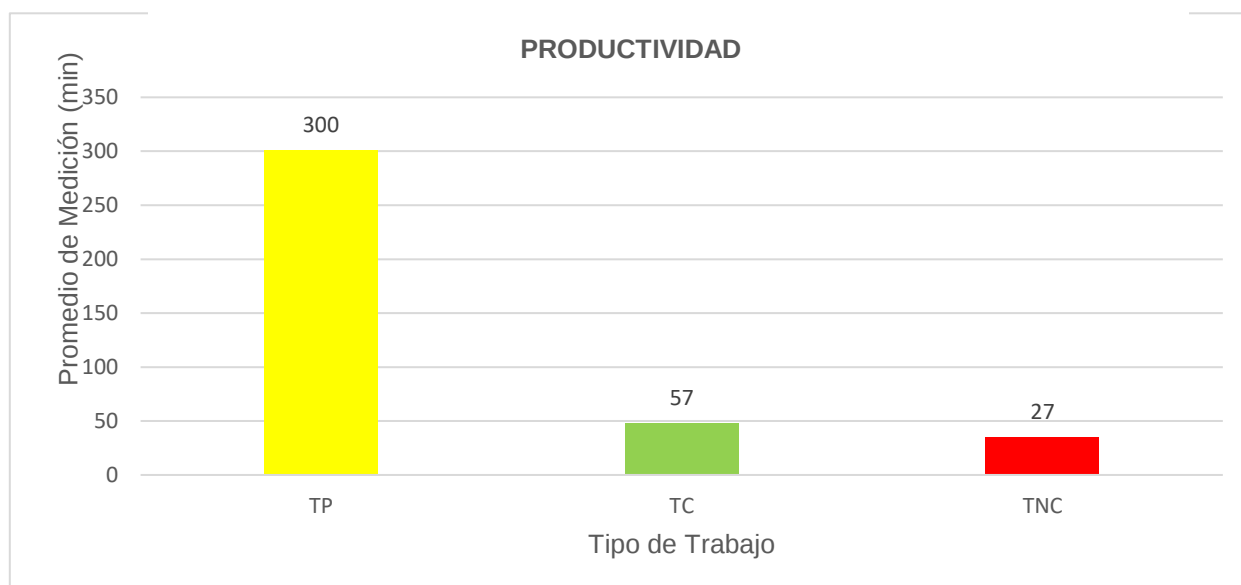
Gráfico 17: Promedio de Medición (min) Vs Tipo de Trabajo - Partidas de Encofrado y Desencofrado
