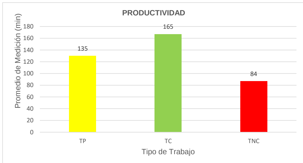
Gráfico 15: Promedio de Medición (min) Vs Tipo de Trabajo - Partidas de Concreto f'c = 210 \text{ kg/cm}^2
