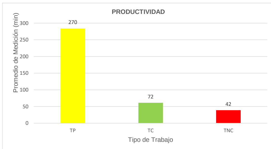
Gráfico 16: Promedio de Medición (min) Vs Tipo de Trabajo - Partidas de Acero de Refuerzo f_y = 4,200 \text{ kg/cm}^2
