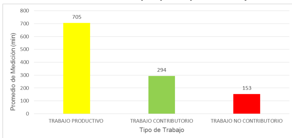
Gráfico 18: Promedio de Medición (min) Vs Tipo de Trabajo Consolidado
