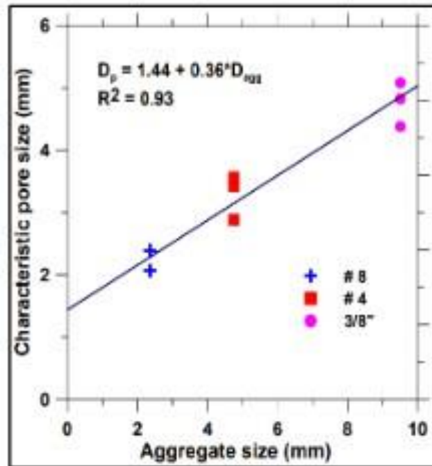
Ilustración 13: Influencia del tamaño del agregado grueso en el tamaño del poro en las mezclas de concreto permeable de un solo tamaño de agregado
