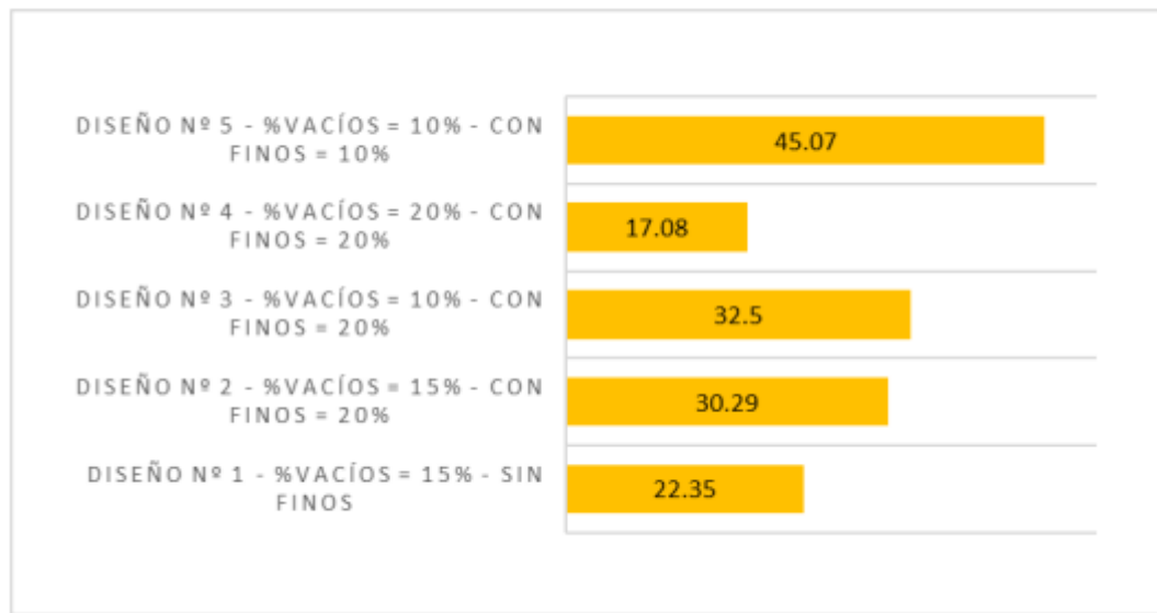
Ilustración 24: Resultados de Resistencia a la Flexión
