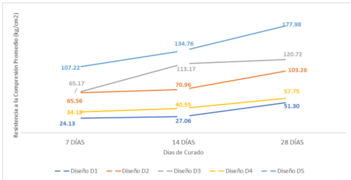
Gráfico 2: Resistencia a la Compresión Promedio con respecto a los días de curado
