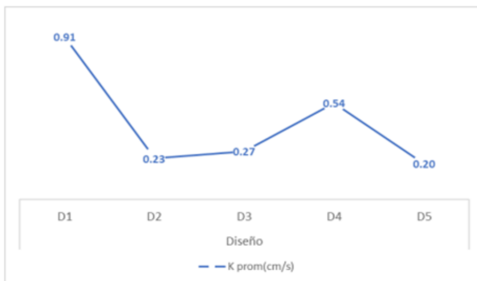
Ilustración 21: Permeabilidad promedio con respecto al diseño de especímenes
