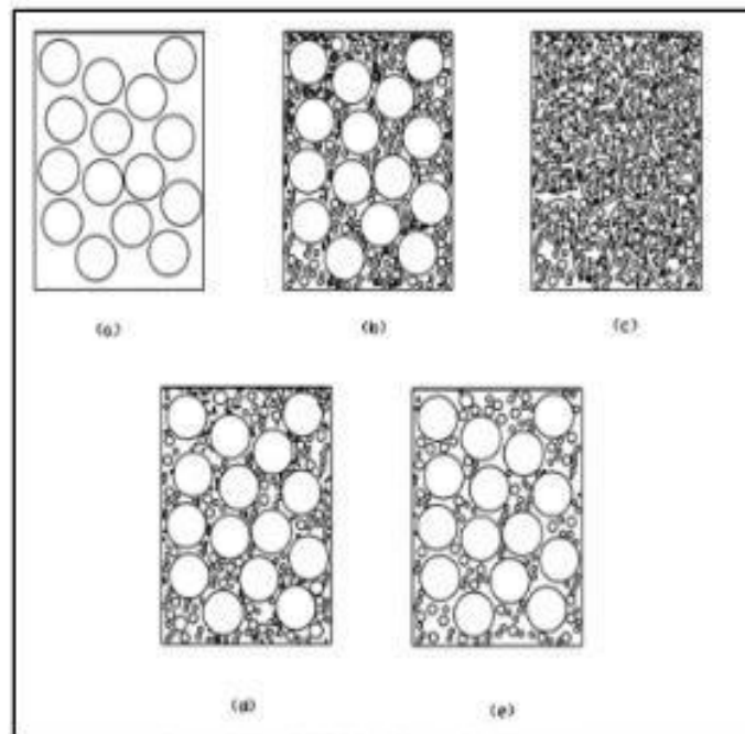
Ilustración 16: Representación esquemática de la granulometría de los agregados en un ensamble de agregados: (a) tamaño uniforme, (b) granulometría continua, (c) reemplazo de partículas pequeñas por partículas grandes, (d) granulometría discontinua, (e) granulometría
