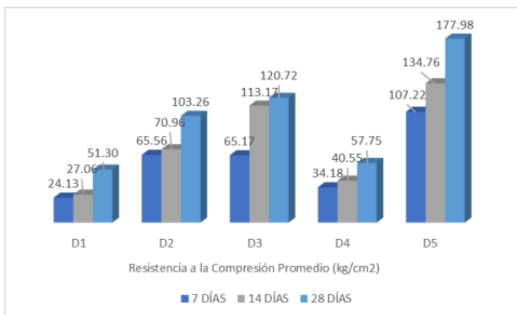
Gráfico 1: Resistencia a la Compresión Promedio con respecto a los diseños
