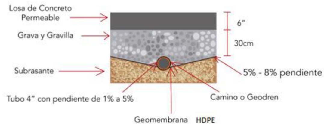
Ilustración 22: Propuesta de Pavimento Propuesto
