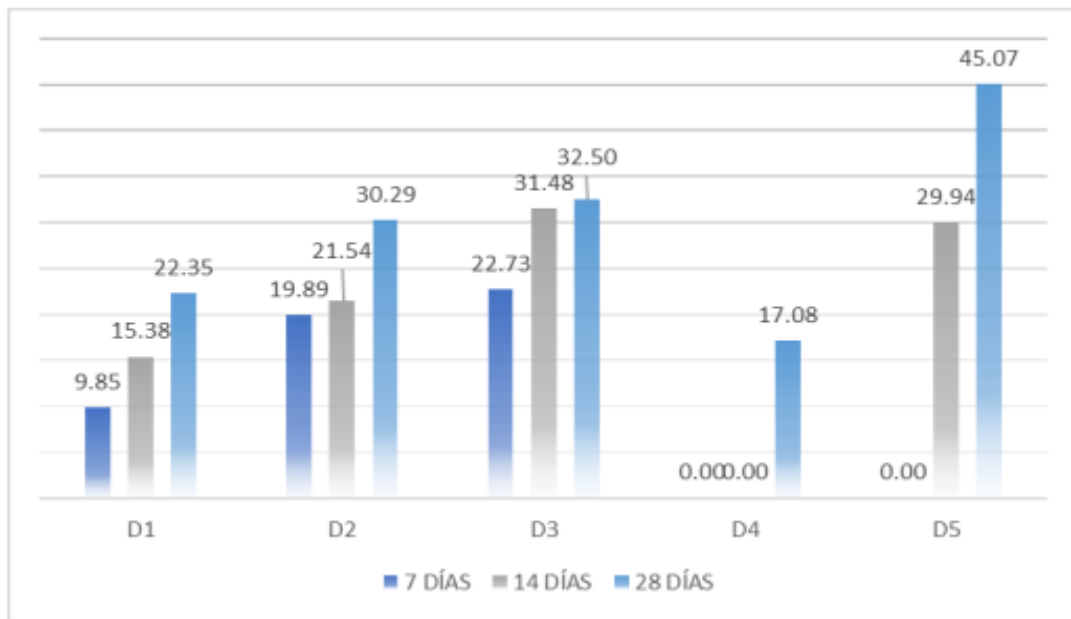
Ilustración 20: Resistencia a la Compresión Promedio con respecto a los diseños
