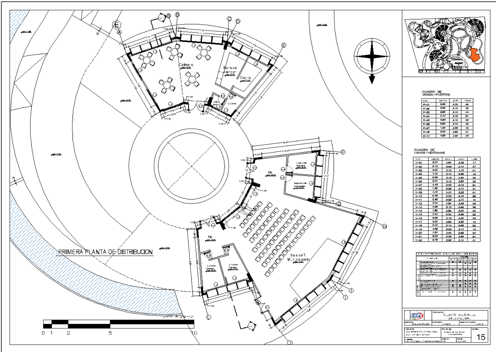
LÁMINA 23. PLANTAS Y CORTES DEL MÓDULO E
