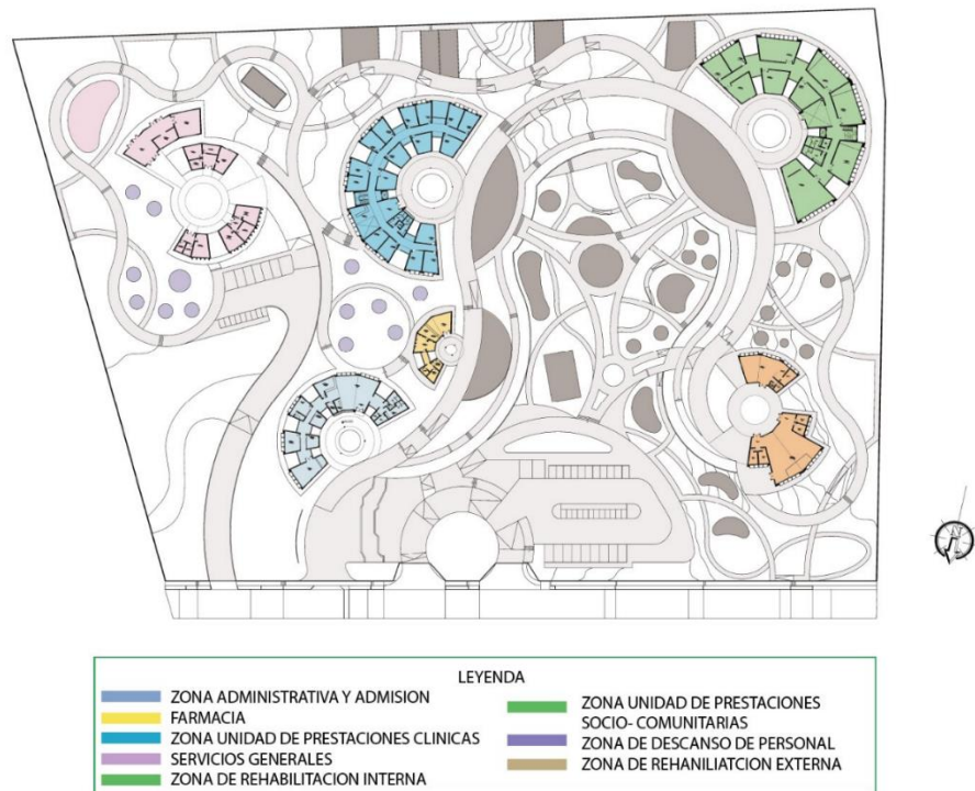
Figura32. Zonificación General
