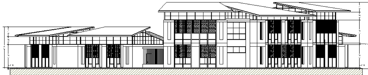
ELEVACION POSTERIOR (MODULO C)
