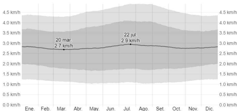
Figura26. Velocidad promedio del viento en Iquitos
