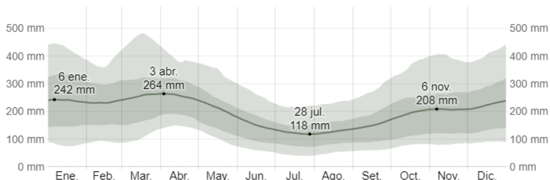
Figura24. Promedio mensual de lluvia en Iquitos
