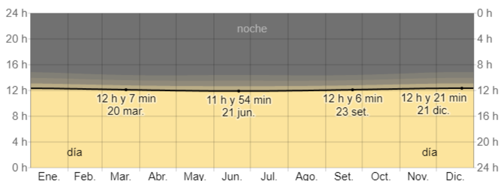
Figura25. Horas de luz natural y crepúsculo en Iquitos
