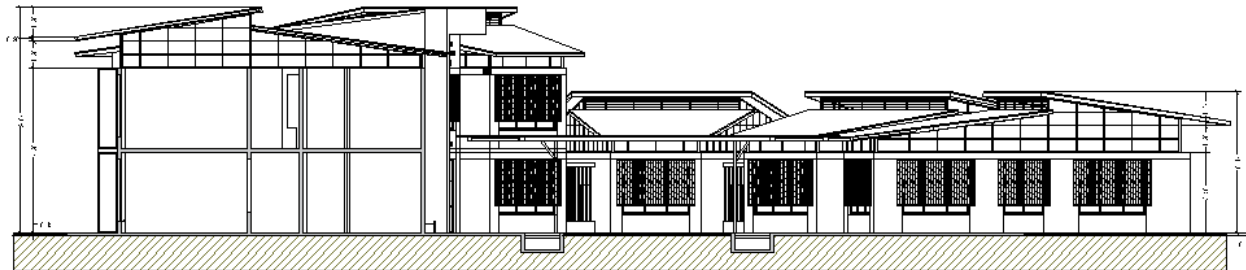
CORTE 1-1 (MODULO C)
