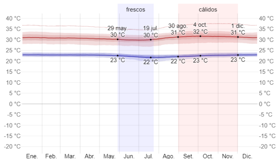
Figura23. Temperatura máxima y mínima promedio en Iquitos
